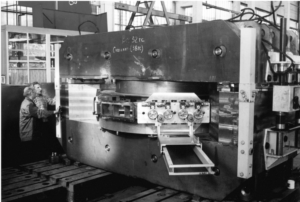
Изохронный циклотрон для промышленного производства трековых мембран
