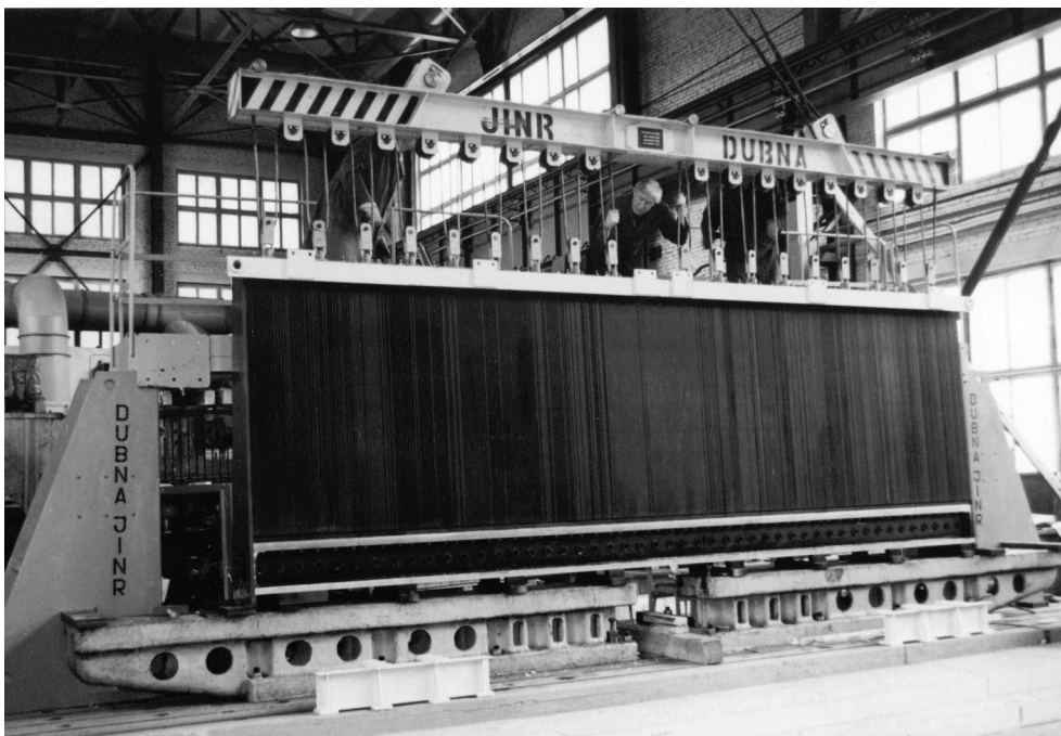
Цех Опытного производства. Сборка модулей детектора ATLAS
