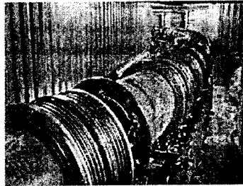
Fig. 1: The Nuclotron.
