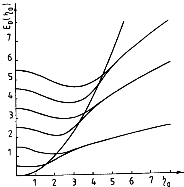
Рис.1. График зависимости высоты барьера и первых шести уровней энергии от параметра \eta_0 .
