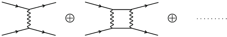
Fig. 6.1 Feynman diagrams
