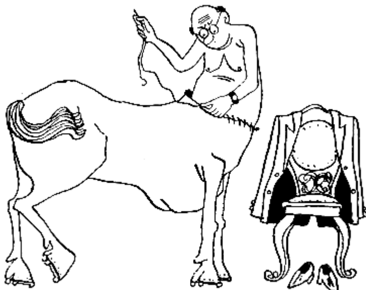
Взаимоисключающие понятия
