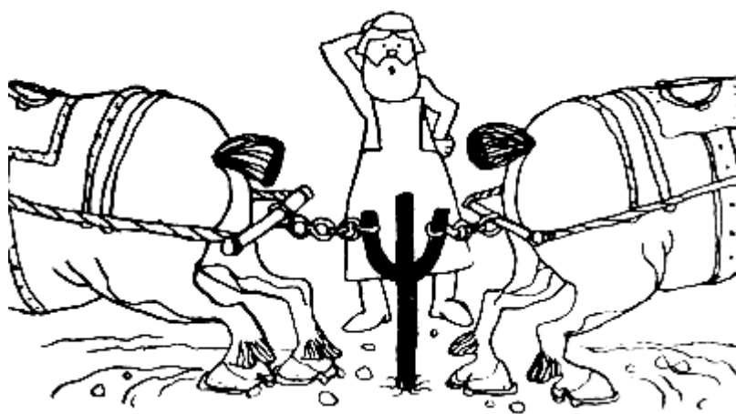
Внутренняя энергия атома
