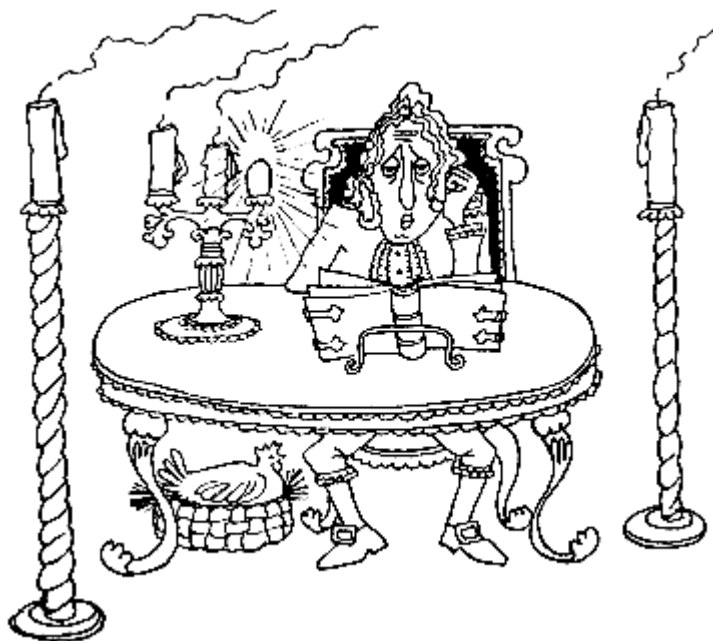
Бенджамен Франклин
