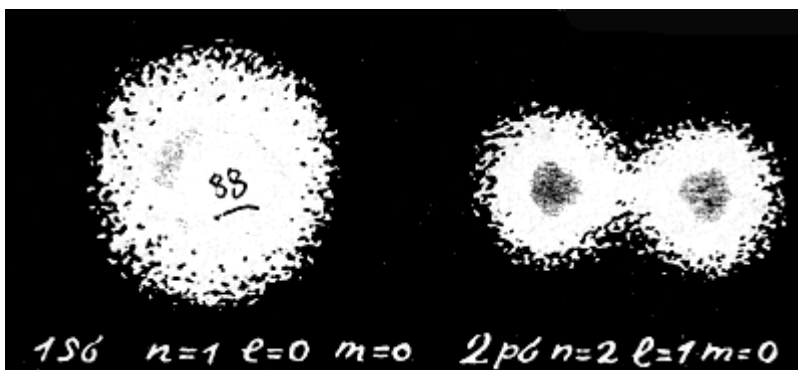
Форма электронного облака 1
