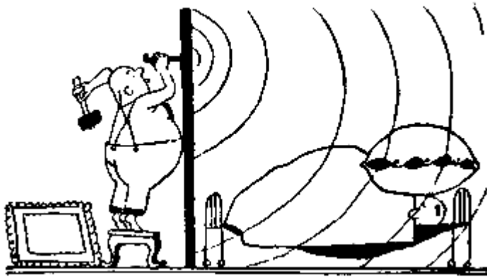
Волны материи
