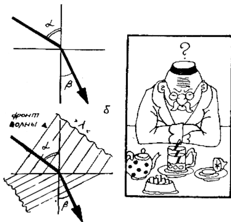
Траектория светового луча
