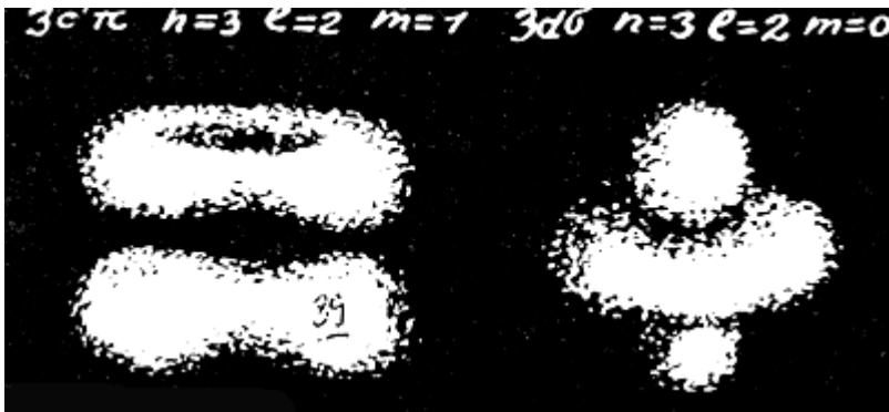
Форма электронного облака 2
