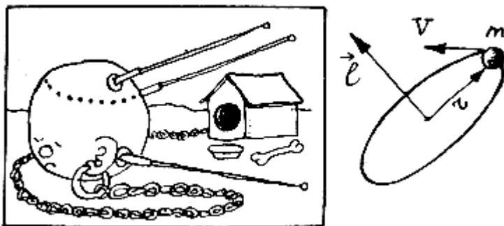
Условие стационарных орбит
