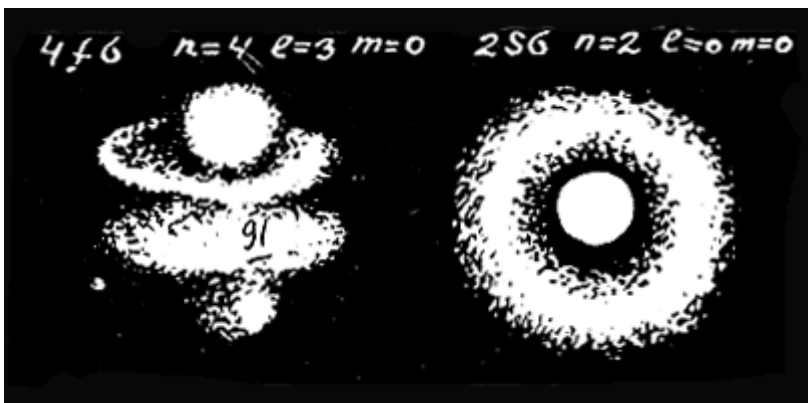
Форма электронного облака 4
