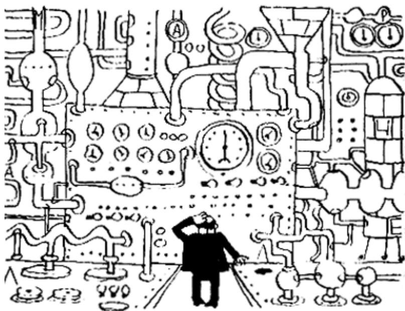
Физическая реальность
