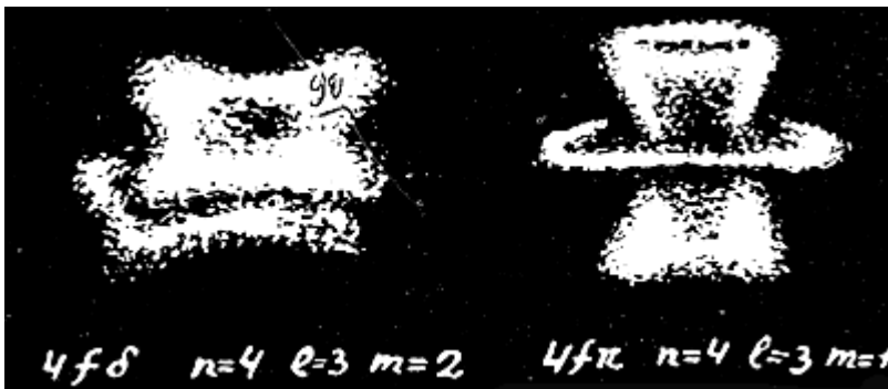
Форма электронного облака 3
