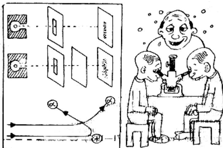
Фольга на пути потока частиц
