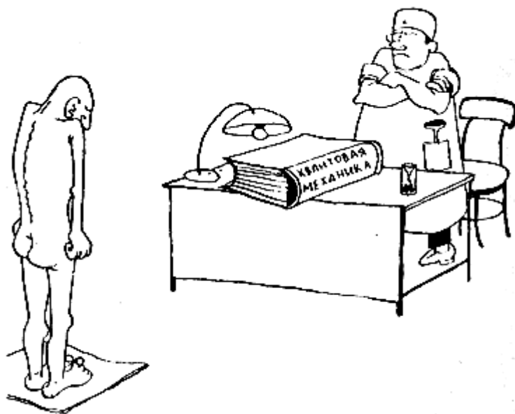
Голые факты
