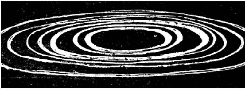
Траектория частицы
