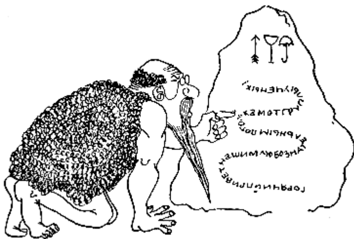
Хаос чисел
