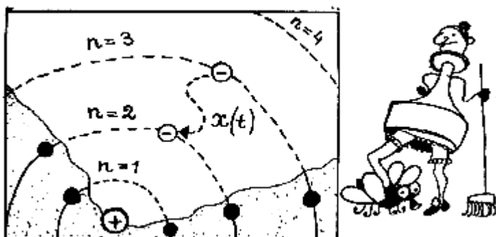
состояние атома в виде бесконечной шахматной доски
