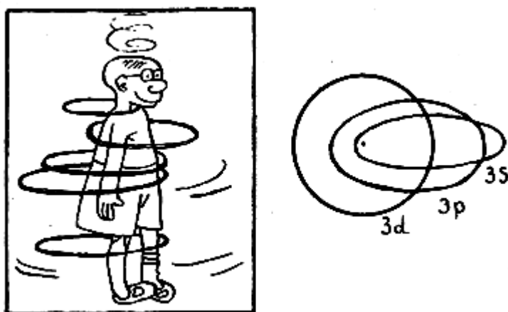
Орбитали
