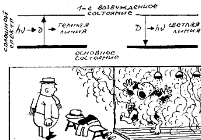
Зоммерфельд
