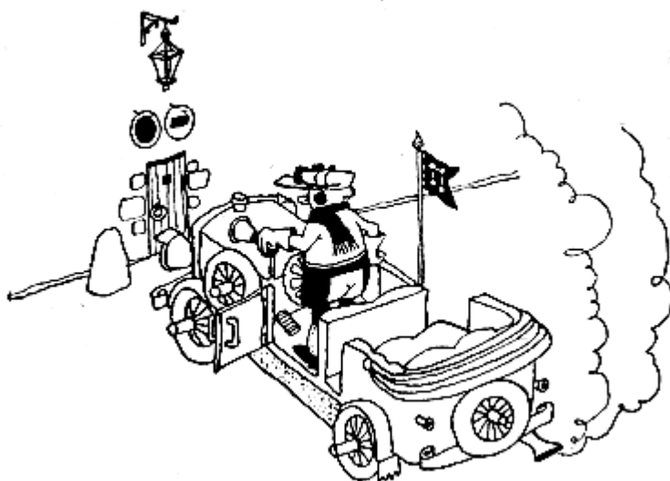
Исследование Резерфорда
