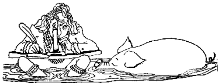
Атомы
