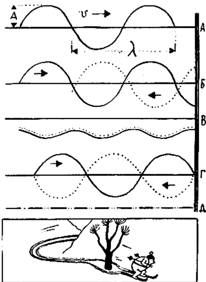
Длины волн
