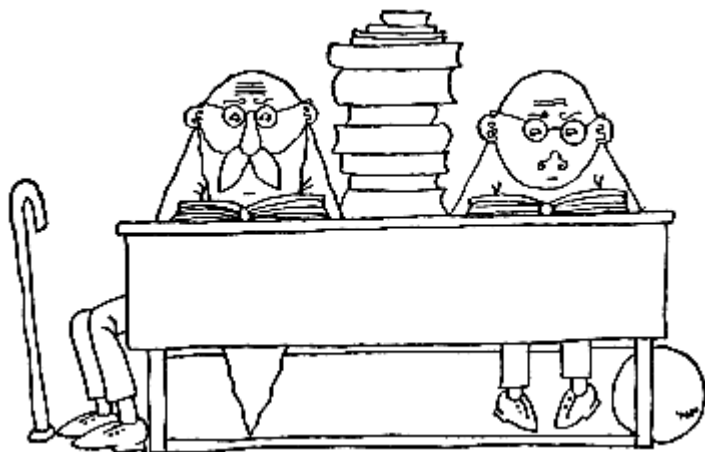
Сомнения
