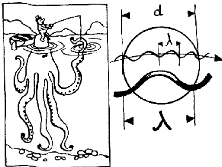
Волновая механика
