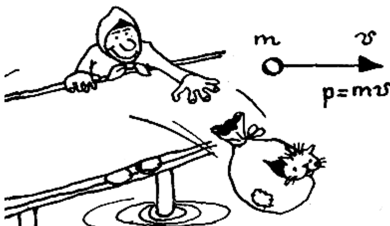
Логическая непротиворечивость
