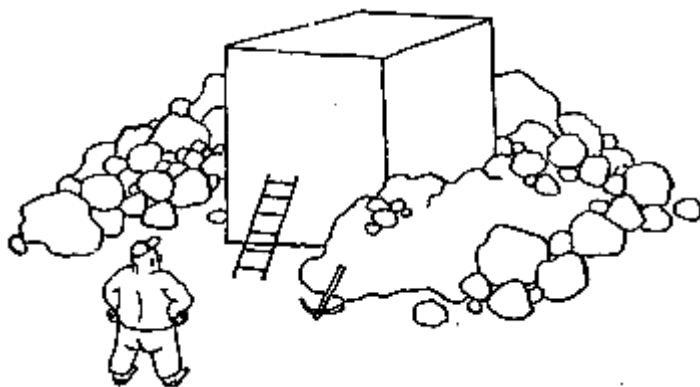
Волны вероятности
