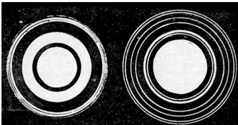
Траектория светового луча
