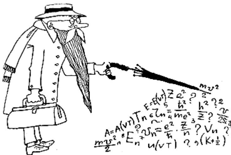
Макс Планк
